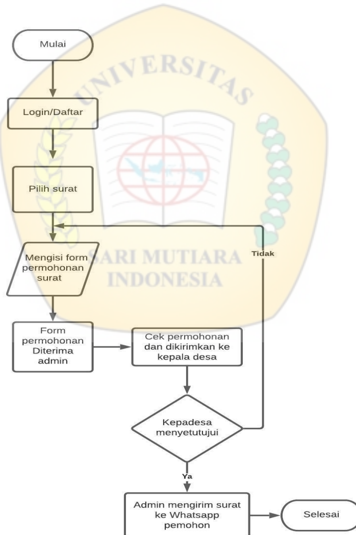
Gambar 3.1 Flowchart Cara Kerja Sistem Mandiri
